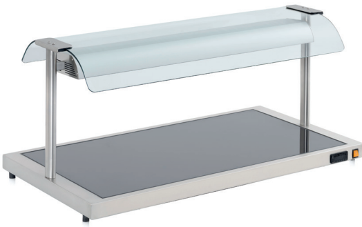
Set Üstü Sıcak Teşhir 3 GN Carving 3 GN
