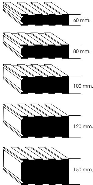
Soğuk Oda Panel Kalınlıkları Cold room panel thicknesses
